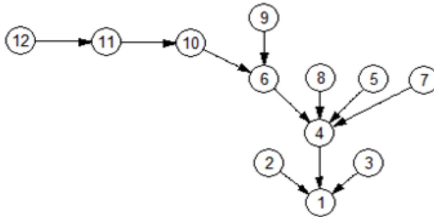
Рисунок 1 – Орграф G информационной структуры модуля системы климата
