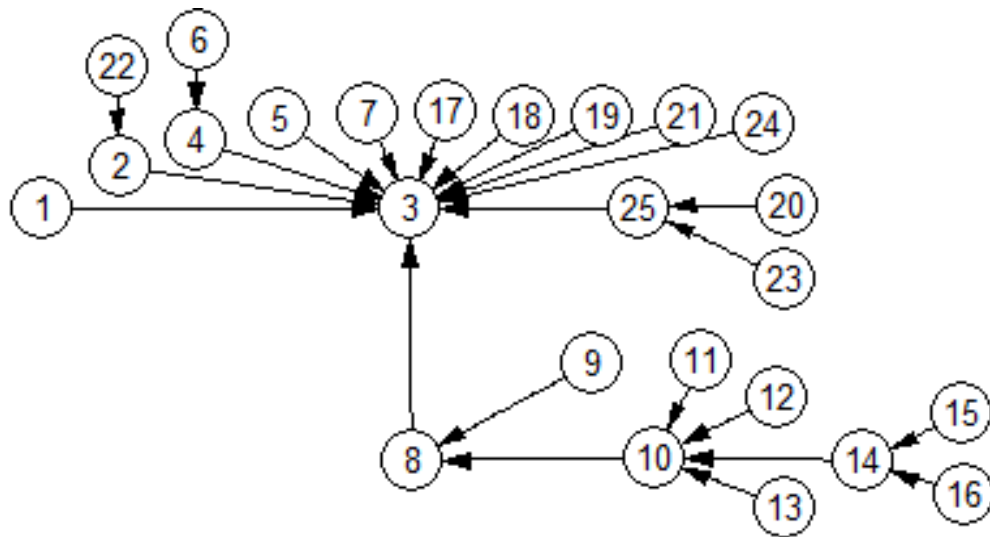
Рисунок 1 – Орграф G информационной структуры модуля управления
