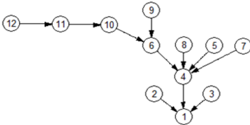
Рисунок 1 – Орграф G информационной структуры модуля бытовых приборов
